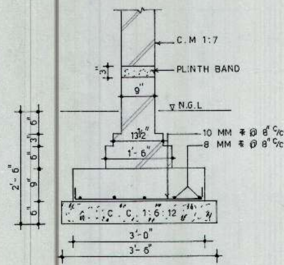
WALL W-3
