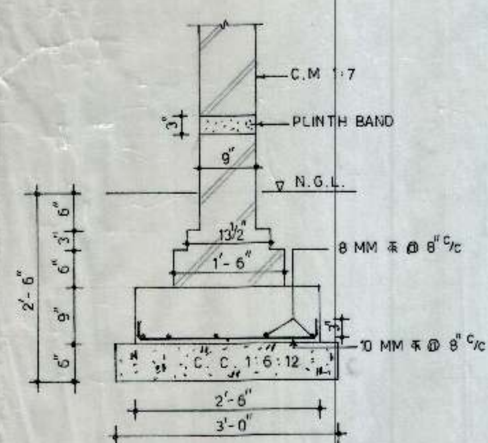
WALL W-1
