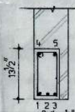
LINTEL L-3
