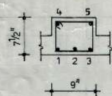
BEAM B-101
