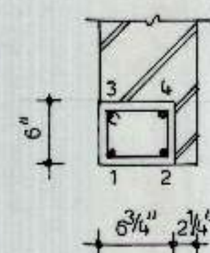
LINTEL L-101
