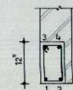
LINTEL L-2
