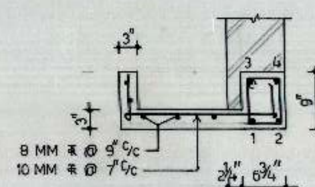
LINTEL L-1
